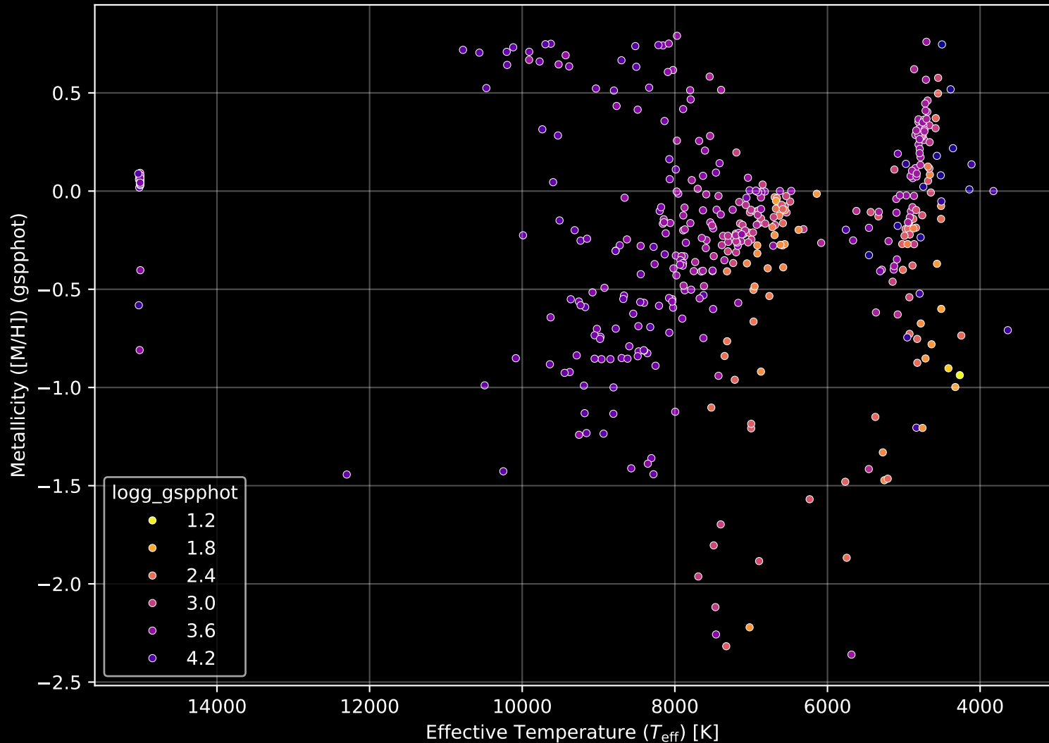
APOGEE DR17 Field: [259+00] Stellar Population Parameters (n= 455)
